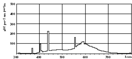
TL- E Circular/33- 640
