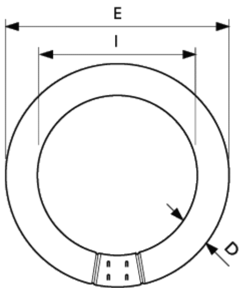
TL- E Circular
