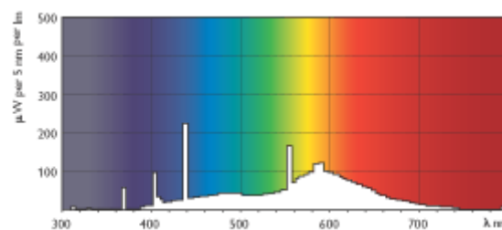
TL- E Circular/33- 640
