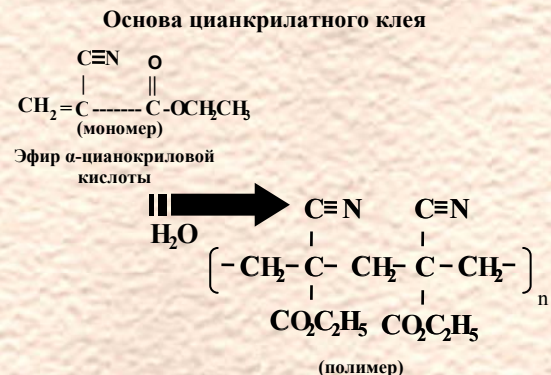
Рис. 1. Схема полимеризации эфира α-цианакриловой кислоты
